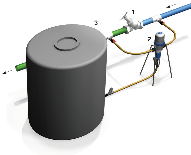
Typowa instalacja obejściowa dla pojedynczego wtryskiwacza MixRite TF.
